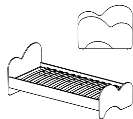
Postel Čelo postele 147101 Korpus 147501 2036x970x770
