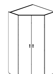
Skřín Korpus 144106 Dveře (1 kus) 145102 1228x1028x2100
