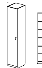
Skřín Korpus 144101 Dveře 145102 410x450x2100
