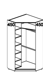
Skřín Korpus 144103 Čelo zásuvky (1 kus) 147602 Dveře (a) 145103 Dveře (b) 145102 820x600x2100
