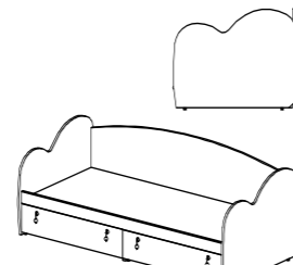
Válenda Válenda 148601 Čelo úložného prostoru (1 kus) 147601 2036x964x795
