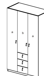
Skřín Korpus 144105 Čelo zásuvky (1 kus) 147602 Dveře (a-1 kus) 145102 Dveře (b-1 kus) 145103 1230x600x2100
