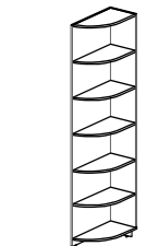
Rohová skřín (zobr.) 144303 Rohová skřín (zrcad.) 144304 300x580x2100
