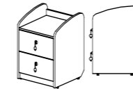
Noční stolek Korpus 142902 Čelo zásuvky (1 kus) 147602 446x450x650
